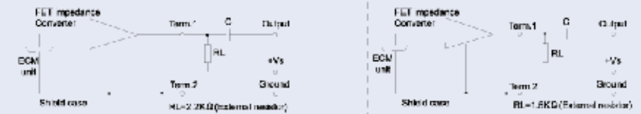
Schematic Diagram 測定電路圖
