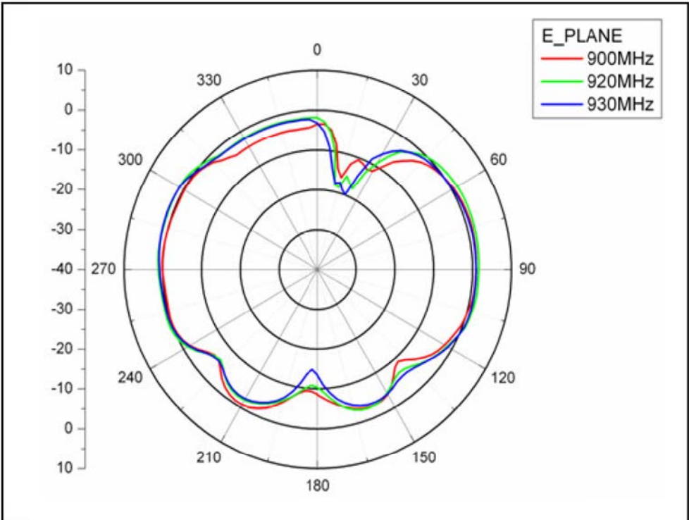
E-plane
