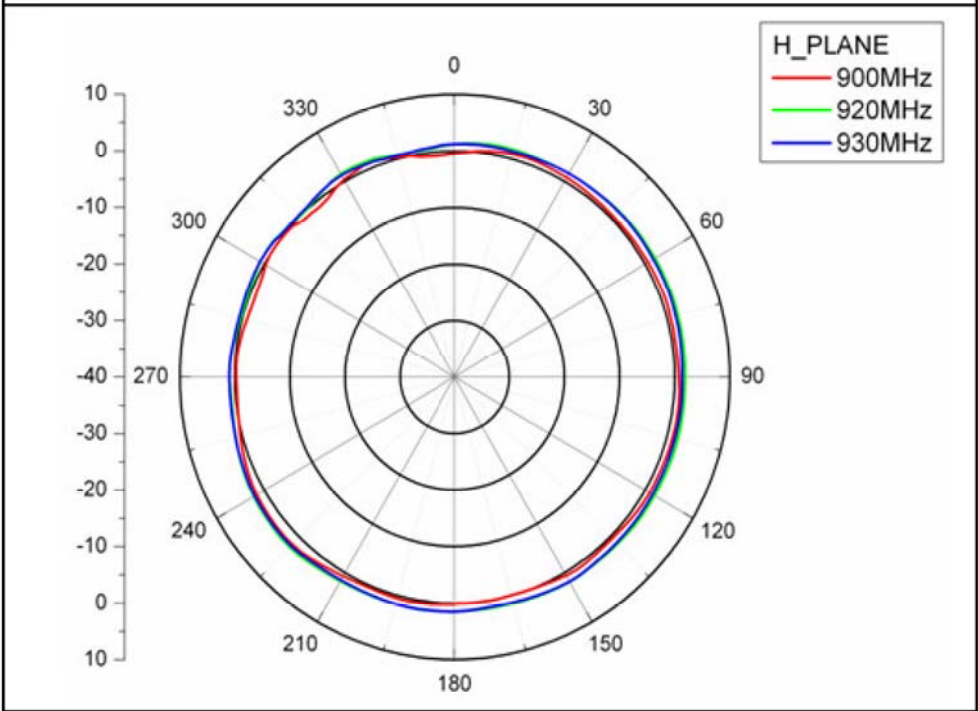
H-plane
